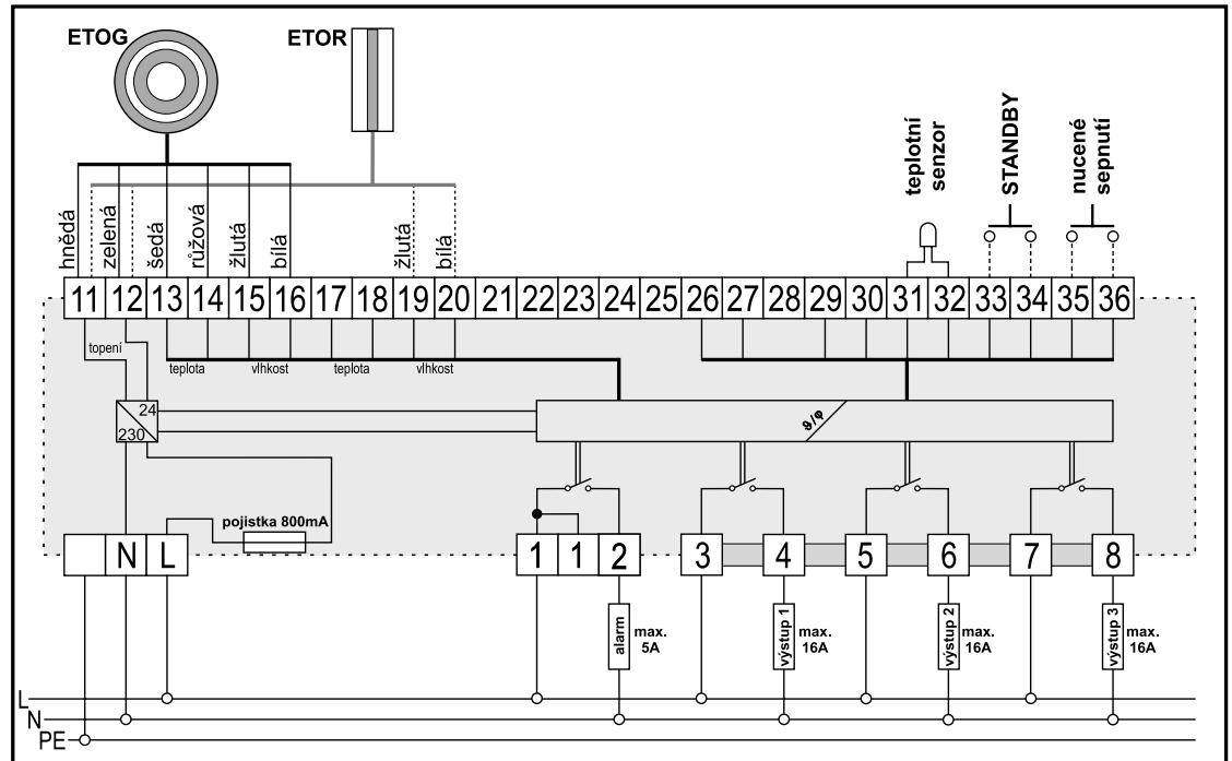
schéma zapojení ETO2 s čidlem ETOG, ETOR a s teplotním senzorem
