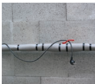
zakrytí topného kabelu izolací
