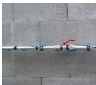
instalace topného kabelu PPC na potrubí
